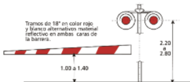
Barreras Ferroviarias
